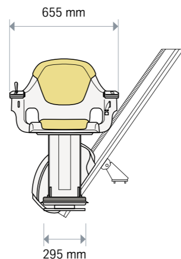
Vista frontale montascale a poltroncina
