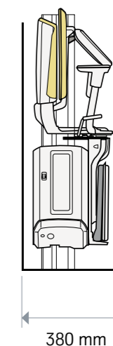
Vista frontale - montascale chiuso
