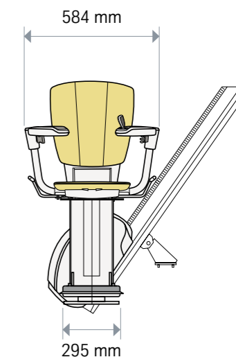
Vista frontale montascale a poltroncina
