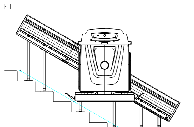
Vista frontale montascale a piattaforma
