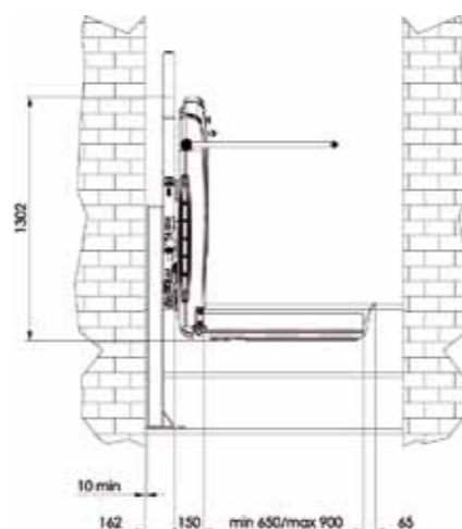
Vista laterale - piattaforma aperta
