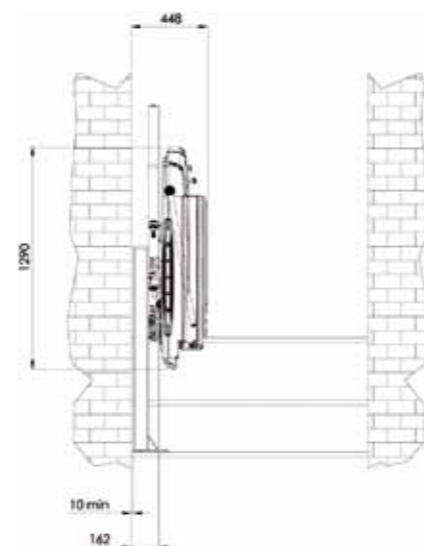
Vista laterale - piattaforma chiusa
